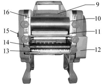
Рис 2: Вид спереди
